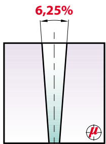
TAPER 6,25% 1:16 CONICIDAD 銜度
